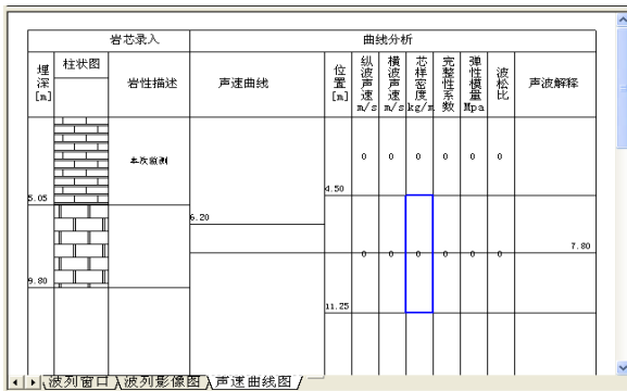
图 7.12 波速直方图
